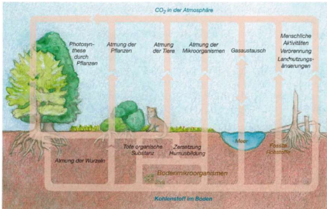
Eenvoudige voorstelling van de bekendste elementen in de koolstofcyclus
